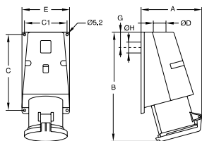
Ölçüler (mm)
