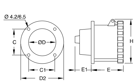
Ölçüler (mm)
