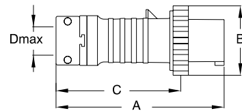
Ölçüler (mm)
