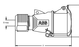
Ölçüler (mm)
