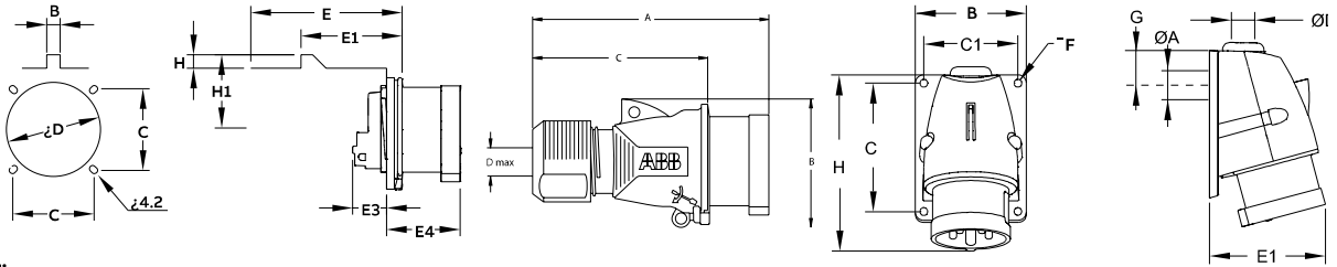
Ölçüler (mm)
