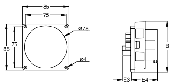
Ölçüler (mm)
