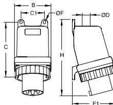
Ölçüler (mm)
