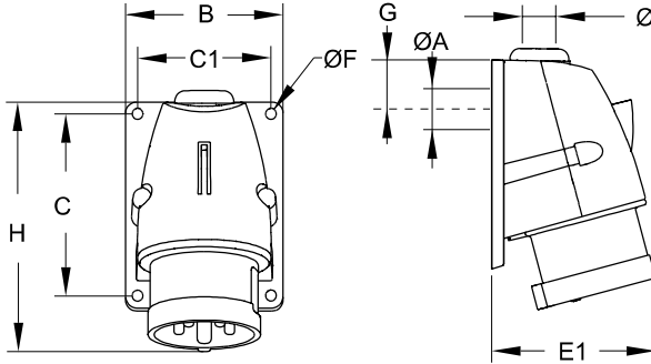
Ölçüler (mm)
