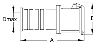
Ölçüler (mm)
