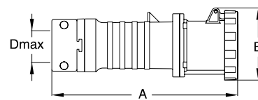
Ölçüler (mm)
