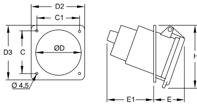
Ölçüler (mm)
