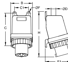
Ölçüler (mm)
