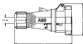
Ölçüler (mm)
