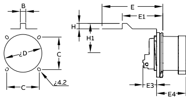
Ölçüler (mm)
